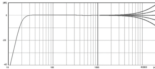
Illustration 6 : Égaliseur ROOM EQ >6 kHz pour les hautes fréquences supérieures à 6 kHz
