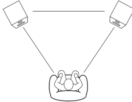
Illustration 2 : Triangle stéréo
