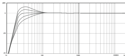
Illustration 7 : Égaliseur ROOM EQ <150 Hz pour les basses fréquences inférieures à 150 Hz
