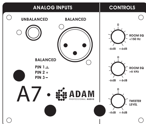
Illustration 4 : Entrées : RCA (asymétrique) et XLR (symétrique) Réglages : Room EQ < 150 Hz, Room EQ > 6 kHz et Tweeter Level
