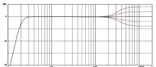
Illustration 5 : Niveau des hautes fréquences
